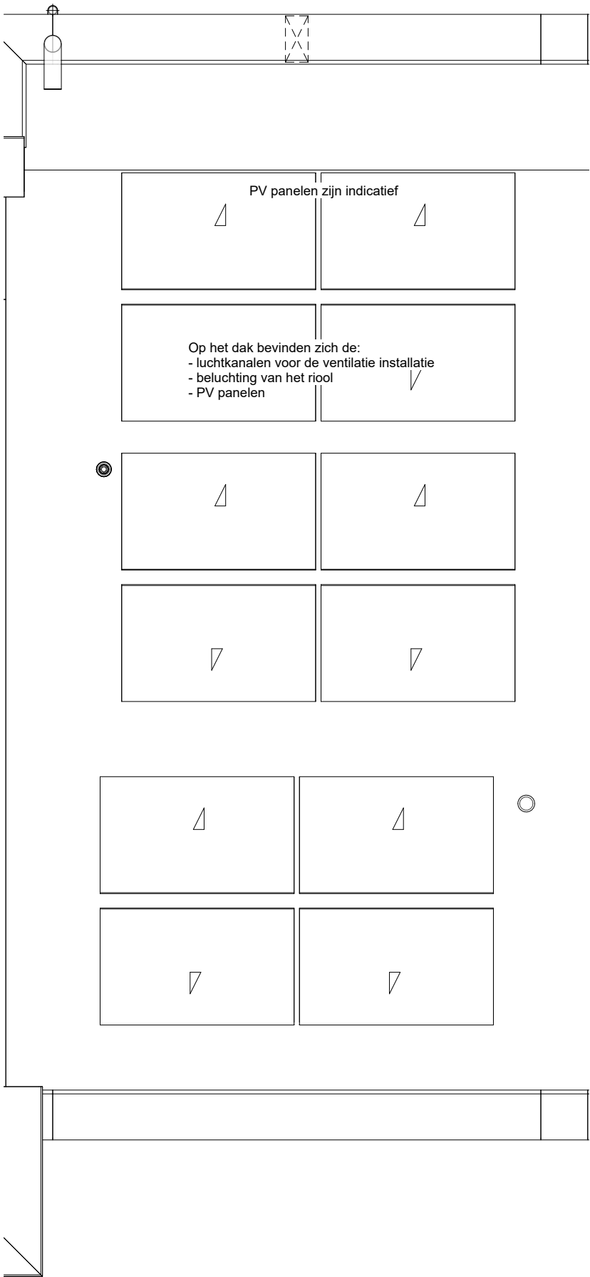
dakaanzicht
