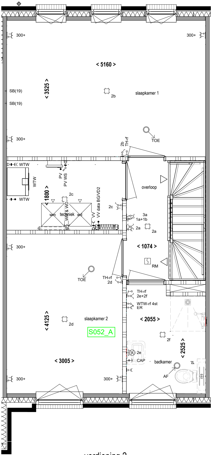
verdieping 2
