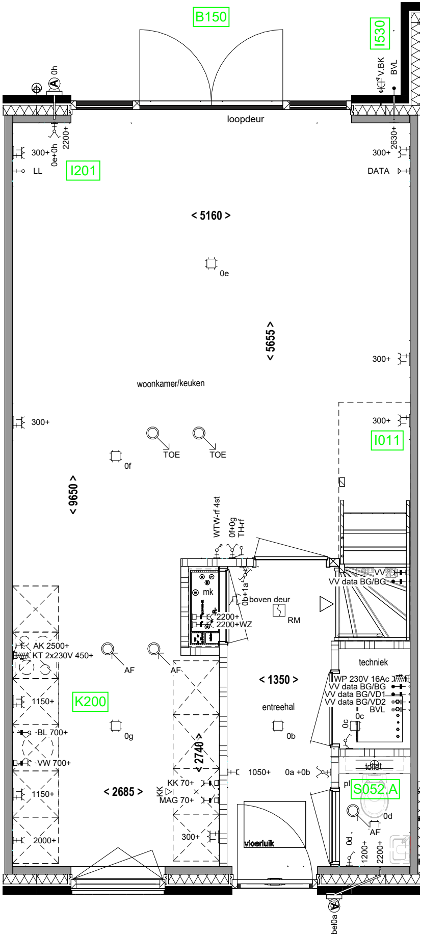
begane grond
