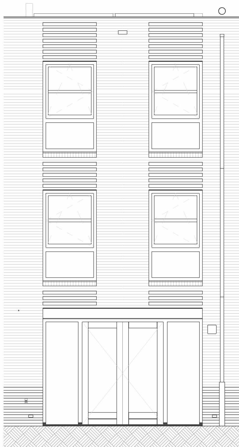
achtergevel
